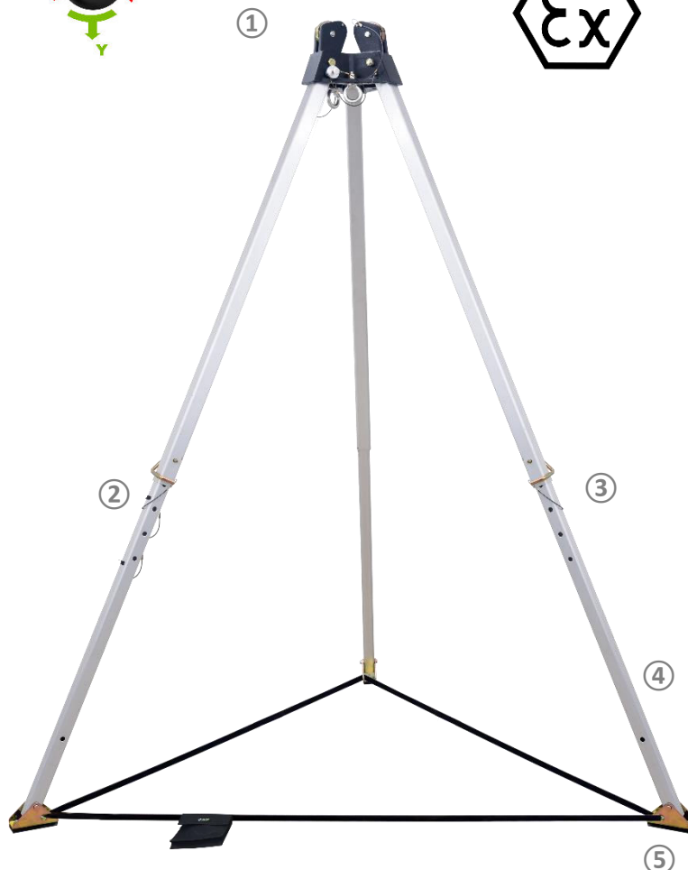
① x2 EN 795 x2 pulleys
